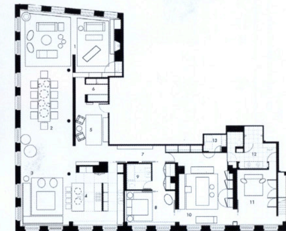
평면도
